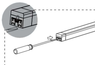
3. Mit Werkzeug den Verbinder öffnen
